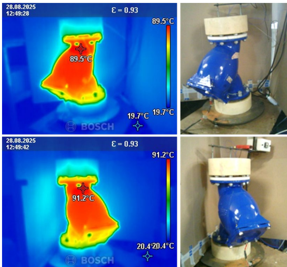
Figur 13: Termografi af testinstallationen samt tilsvarende billede i synligt lys.
