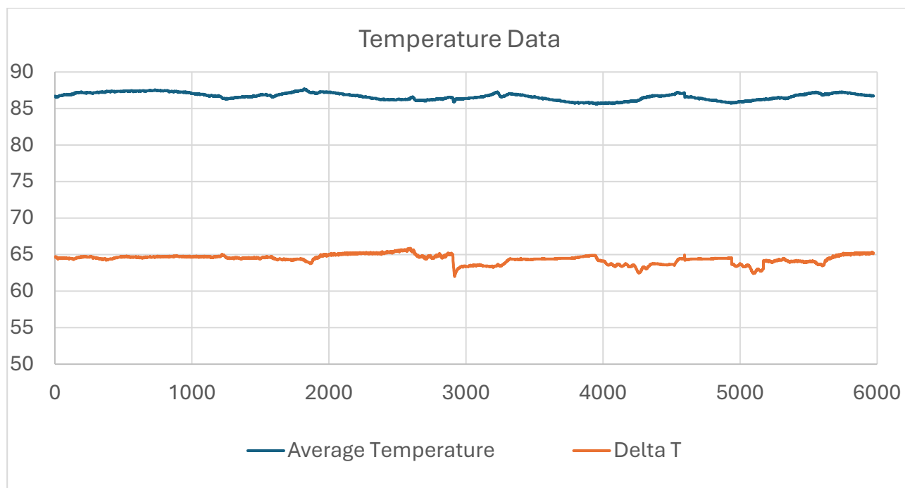
Figur 12: Temperaturdata fra test 1. Y-akse: Temperatur i °C. X-akse: Tid i minutter.
