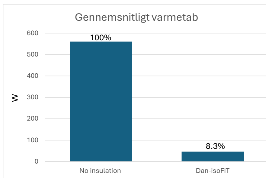
Figure 17: Gennemsnitligt varmetab, mineraluldisolering vs. Dan-isoFIT.
